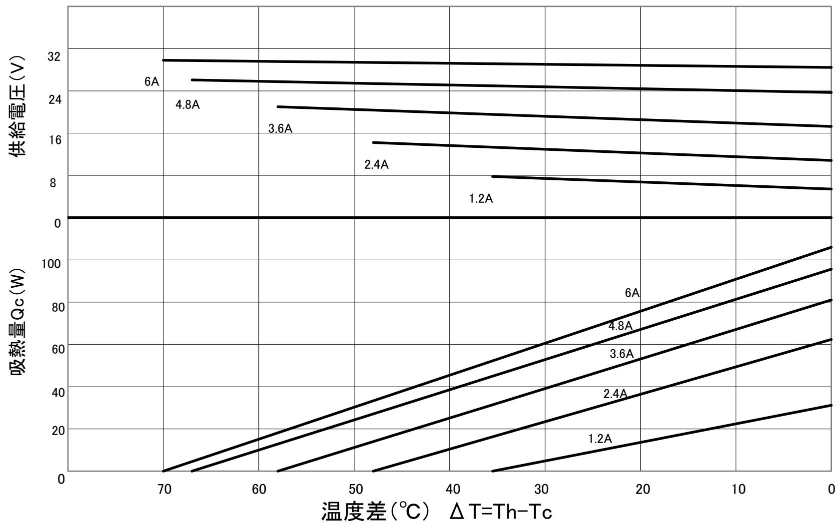
FPH1-24107BC 特性図 (Th=27°C)
