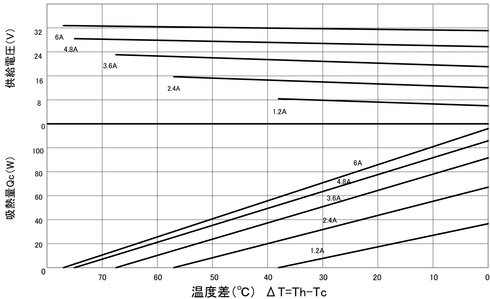
FPH1-24107BC特性図(Th=50°C)
