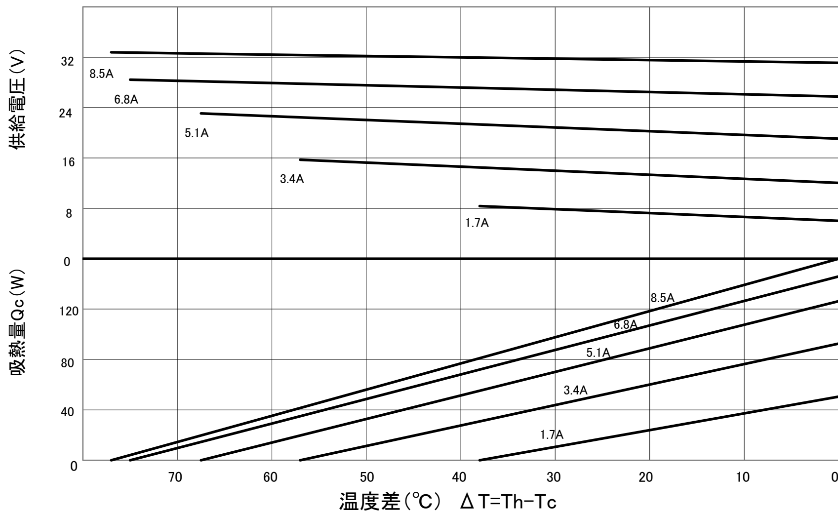
FPH1-24108BC特性図(Th=50°C)
